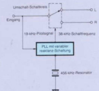
Abb. 5 Stereodemodulator des T-108
