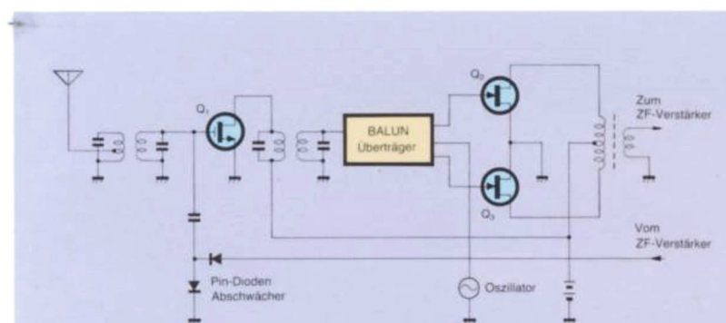
Abb. 1 Schaltbild der Eingangsstufe
