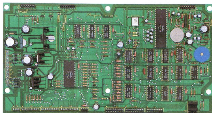
● Logikschaltung mit UKW/MW-Synthesizer, Funktionsspeicher und Pulsabstimmung
