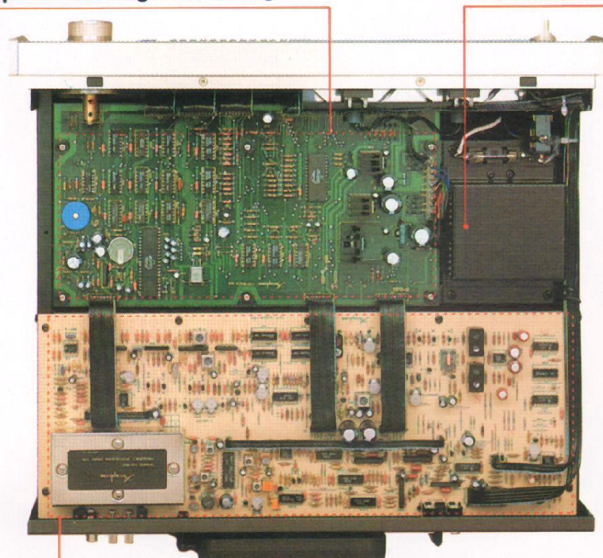
UKW/MW-Tuner-Leiterplatte
