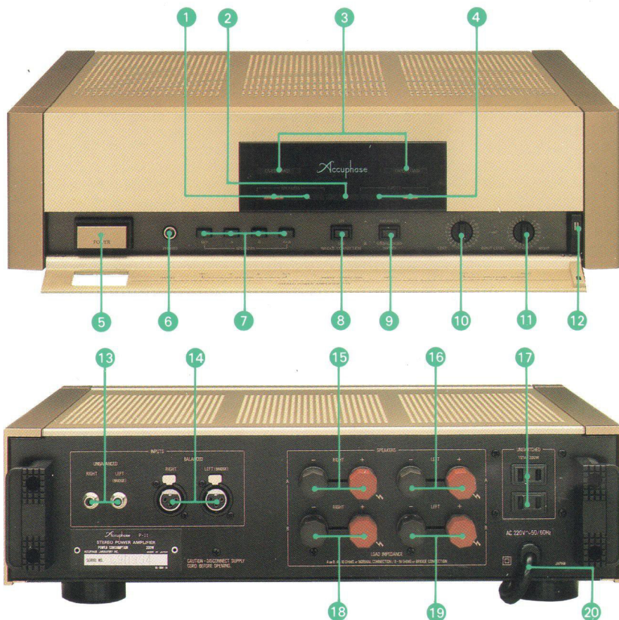
P-11 Frontplatte/Rückwand
