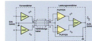
Abb. 2 Prinzip der symmetrischen Signalübergang
