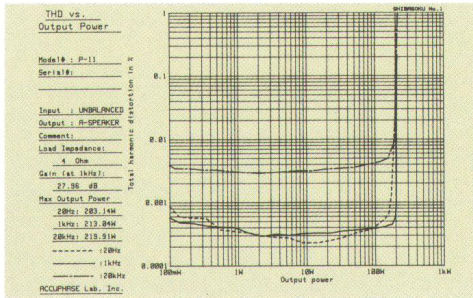
● P-11 Ausgangsleistung gegen Gesamtklirrfaktor (4Ω Belastung, Stereobetrieb)
