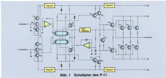
Abb. 1 Schaltplan des P-11
