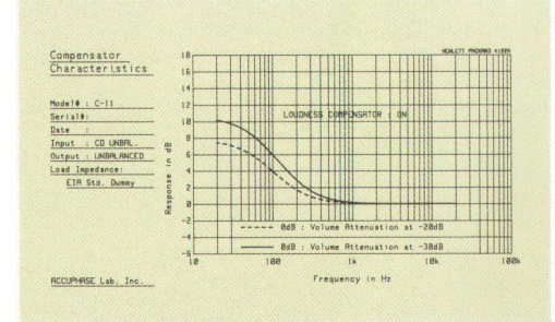
● C-11 Kompensator-Eigenschaften
