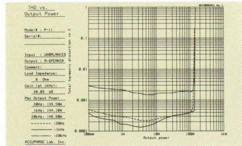
● P-11 Ausgangsleistung gegen Gesamtklirrfaktor (8Ω Belastung, Stereobetrieb)
