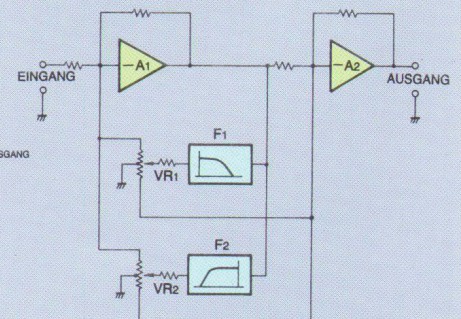
Abb. 5 Schaltkreis der Klangregler (Summier-Filterprinzip)
