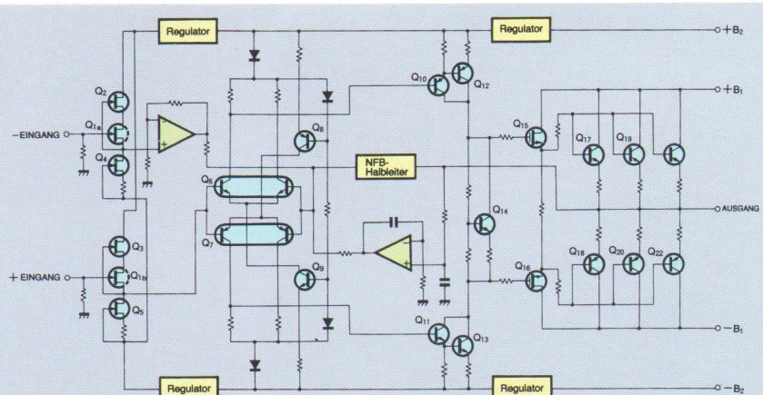
Abb. 1 Schaltplan des P-11
