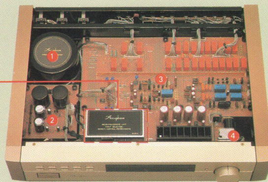
Interne Anordnung
