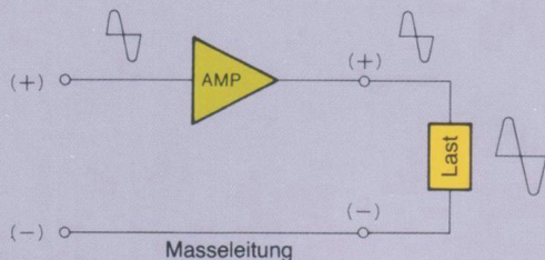
(a) Unsymmetrische Signalübertragung
