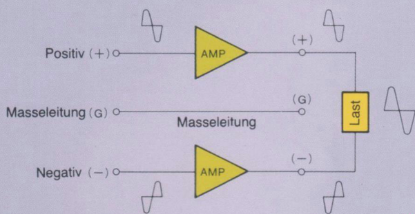
(b) Symmetrische Signalübertragung
