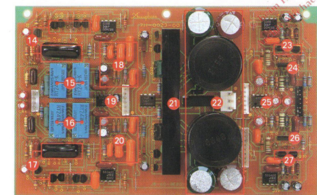
Leiterplatte des Vorverstärkers
