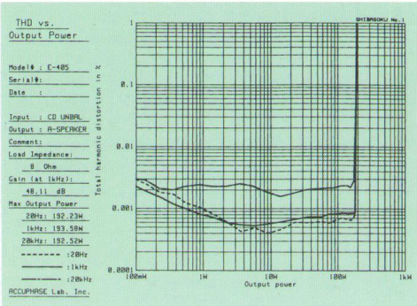
● Ausgangsleistung im Verhältnis zum Gesamtklirrfaktor (THD) (8Ω-Belastung)
