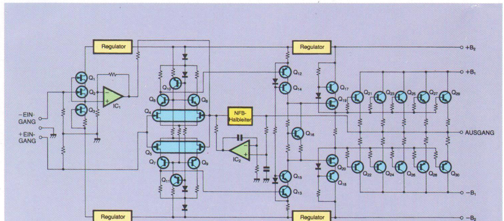
Abb. 1 Schaltplan für den Leistungsverstärker
