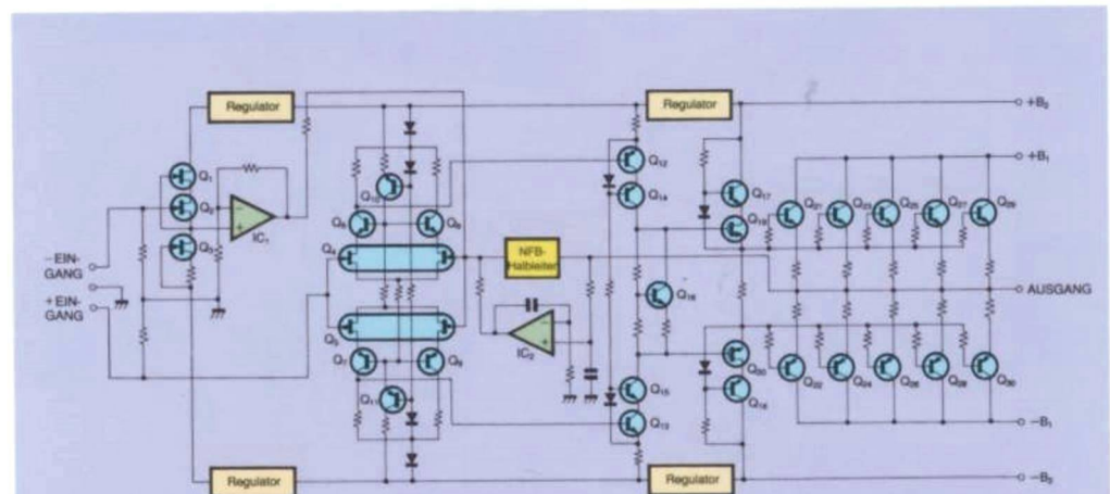
Abb. 1 Schaltplan für den Leistungsverstärker
