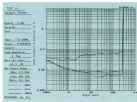
● Ausgangsleistung im Verhältnis zum Gesamtklirrfaktor (THD) (4Ω-Belastung)
