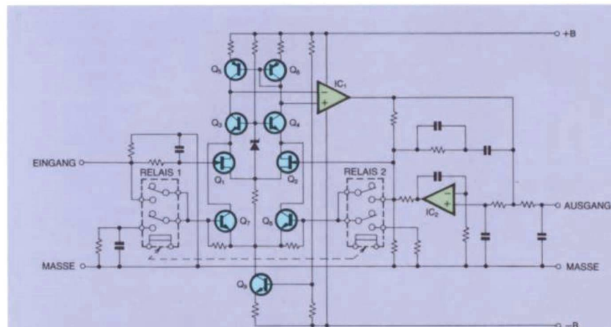
Abb. 3 Schaltplan für den Entzerrer-Verstärker
