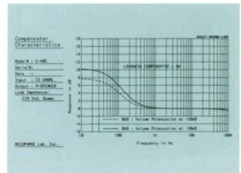
● Kompensations-Eigenschaften
