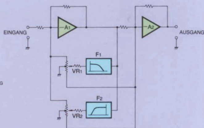
Abb. 4 Beispiel für eine Klangregelungs-Schaltung (durch Summierung der aktiven Filter)
