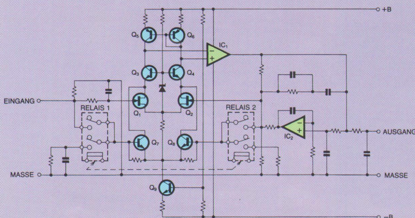
Abb. 3 Schaltplan für den Entzerrer-Verstärker
