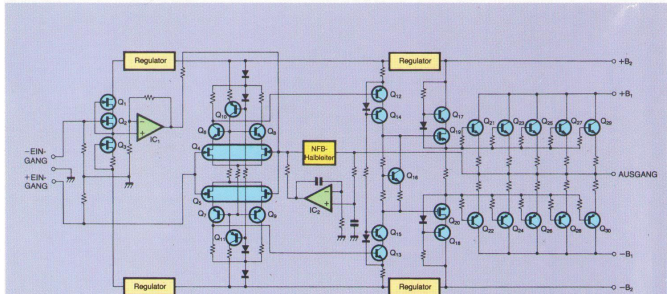
Abb. 1 Schaltplan für den Leistungsverstärker
