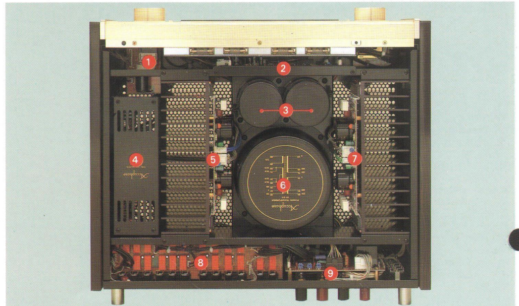
Interne Anordnung
