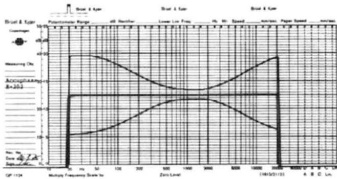
Bild 3 Frequenzgang mit eingeschalteten Klangreglern, gemessen bei 6 dB unter Nennleistung an 8 \Omega
