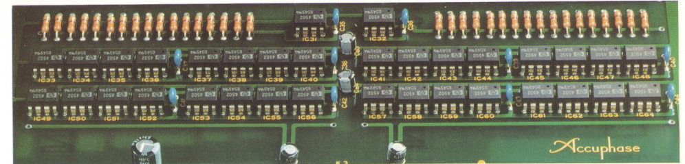
Hochwertige Präzisions-Optokoppler – 17 für jeden Kanal – zur Trennung des digitalen Schaltkreises vom analogen.
