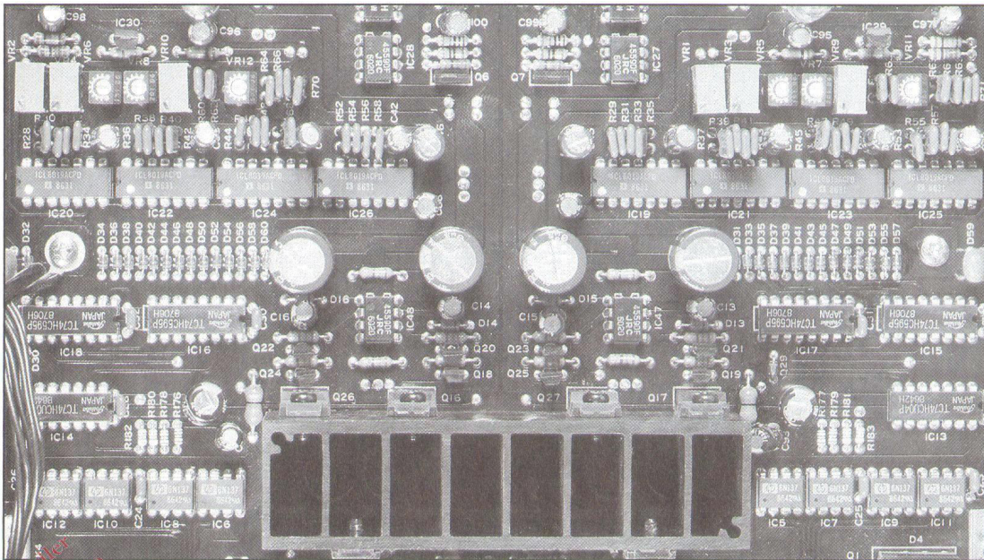
Auf dem oberen Drittel der Wandler-Platine sitzen die Schalter, Widerstände und Digital-Filter des diskret aufgebauten Konverters, rechts und links unten die acht Optokoppler
