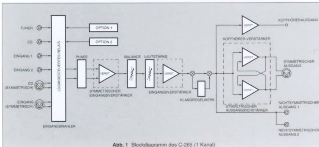
Abb. 1 Blockdiagramm des C-265 (1 Kanal)
