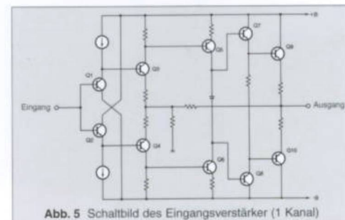
Abb. 5 Schaltbild des Eingangsverstärker (1 Kanal)
