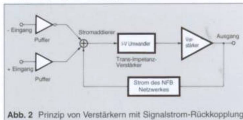
Abb. 2 Prinzip von Verstärkern mit Signalstrom-Rückkopplung
