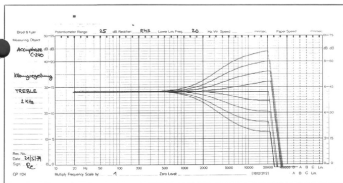
Klangregelung: Treble, Einsatzfrequenz 2 kHz
