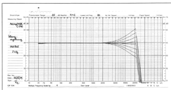
Klangregelung: Treble, Einsatzfrequenz 7 kHz
