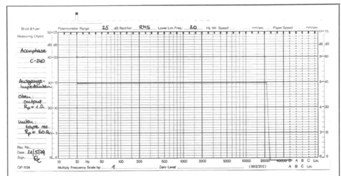
Ausgangs impedanzen; oben: output R_p = 1 Ohm, unten: tape rec. R_p = 60 Ohm
