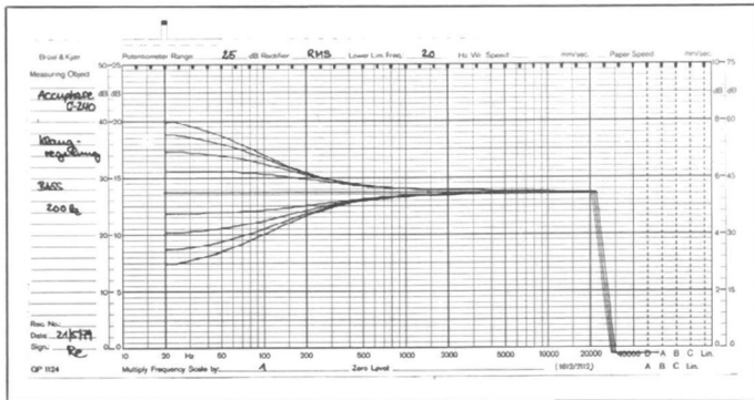
Klangregelung: Bass, Einsatzfrequenz 200 Hz
