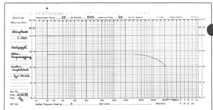
Hochpegel: Frequenzgang und Impedanz
