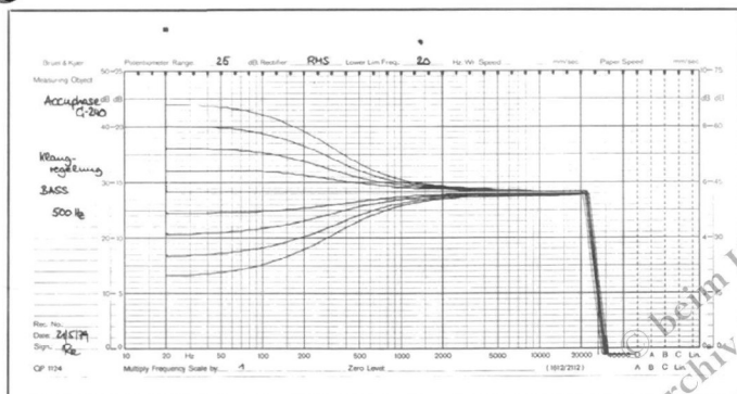
Klangregelung: Bass, Einsatzfrequenz 500 Hz
