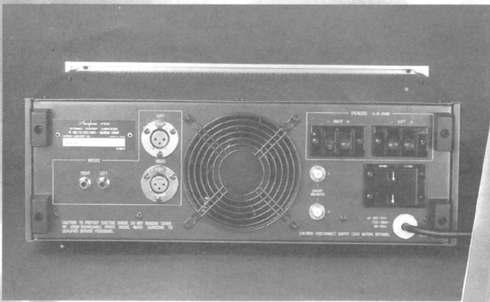
Rückansicht des Accuphase P-400
