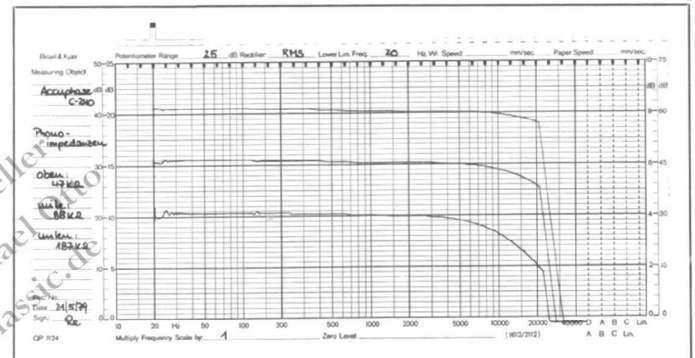
Phonoimpedanzen; oben: 47 kOhm, Mitte: 88 kOhm, unten: 187 kOhm
