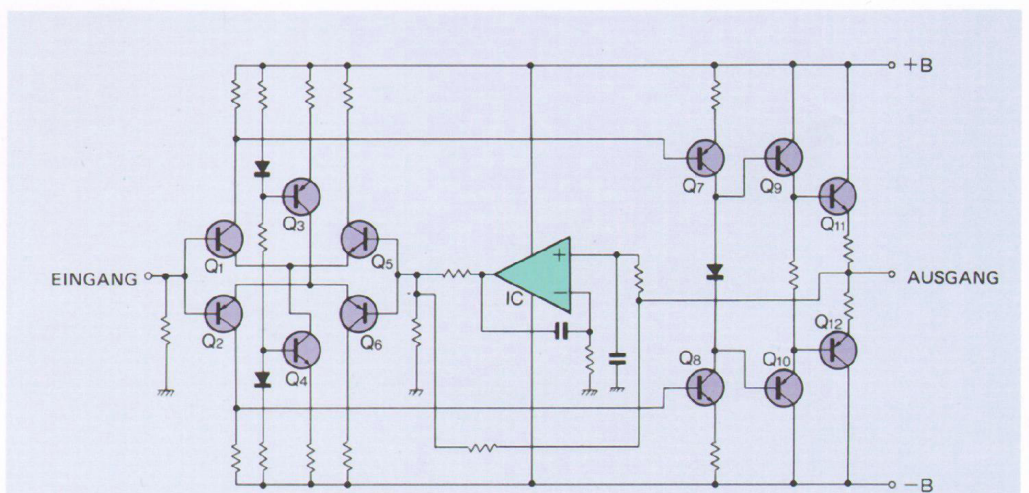
Abb. 1: Schaltplan des Entzerrer- und Hochpegelverstärkers
