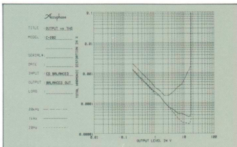
Ausgangsspannung im Verhältnis zum Gesamtklirrfaktor (symmetrischer CD-Eingang, symmetrischer Ausgang)
