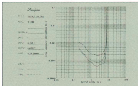
Ausgangsspannung im Verhältnis zum Gesamtklirrfaktor (unsymmetrischer Hochpegeleingang, unsymmetrischer Ausgang)
