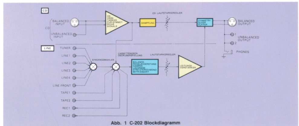
Abb. 1 C-202 Blockdiagramm
