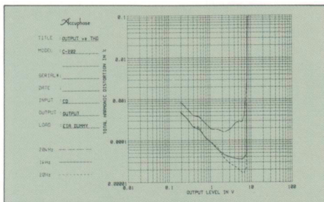
Ausgangsspannung im Verhältnis zum Gesamtklirrfaktor (unsymmetrischer CD-Eingang, unsymmetrischer Ausgang)
