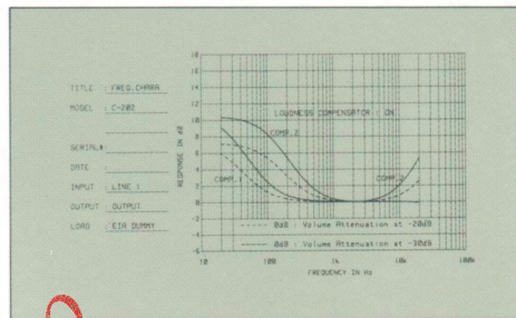
Kompensierter Frequenzgang (unsymmetrischer Hochpegeleingang, unsymmetrischer Ausgang)
