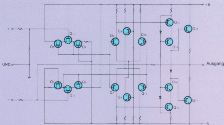
Abb. 2 CD-Verstärkerblock mit symmetrischen Eingängen
