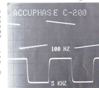
11 Rechteckübertragungsverhalten, aufgenommen mit 4,7 k \Omega Lastwiderstand bei den Impulsfolgefrequenzen 100 Hz und 5 kHz
