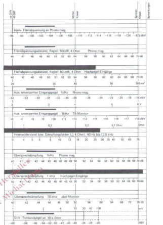
14 Balkendiagramm mit den wichtigsten Leistungsmerkmalen des Endverstärkers P-300
