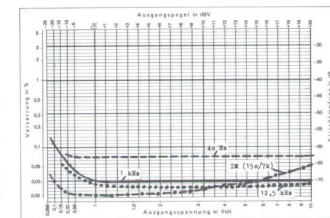
9 Verzerrungsdiagramm des Vorverstärkers C-200, gemessen mit 4,7 k \Omega Abschlußwiderstand
