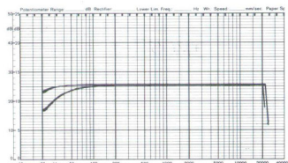
5 Frequenzgang über Eingang Phono, gemessen ohne Verzerter nach RIAA in beiden Kanälen a) ohne Filter b) mit Subsonic-Filter
