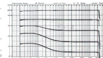
7 Frequenzgang bei gehörigter Lautstärkeregelung (Comp), gemessen bei Nennausgangsspannung in beiden Kanälen und Stellungen des Lautstärkereglers von 0 dB (a) bis -40 dB (e)
