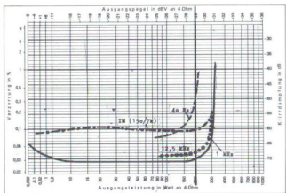
13 Leistung-Verzerrungs-Diagramm des Endverstärkers P-300
