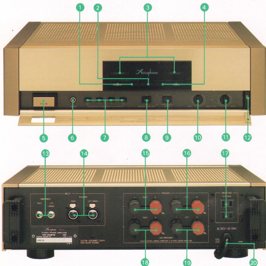
P-11 Frontplatte/Rückwand
