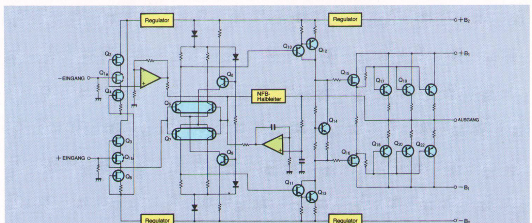
Abb. 1 Schaltplan des P-11
