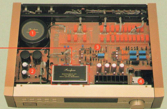
Interne Anordnung
