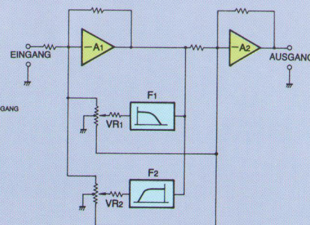
Abb. 5 Schaltkreis der Klangregler (Summier-Filterprinzip)
