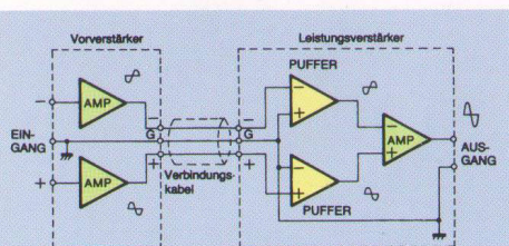
Abb. 2 Prinzip der symmetrischen Signalübergang
