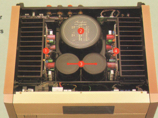
Interne Anordnung
