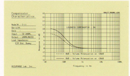
● C-11 Kompensator-Eigenschaften
