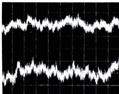
Bild 6a Phonoeingang Vertikal: 50 mV/Div. Horizontal: 5 ms/Div.
