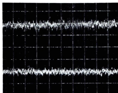
Bild 6b Auxiliary-Eingang Vertikal: 10 mV/Div. Horizontal: 0,5 ms/Div.
