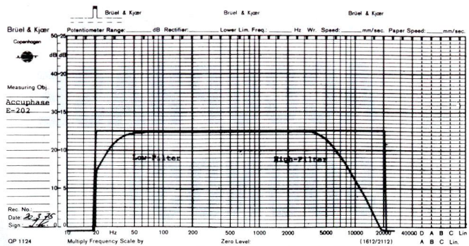
Bild 4 Frequenzgang mit Low- und High-Filter, gemessen bei 6 dB unter Nennleistung an 8 \Omega
