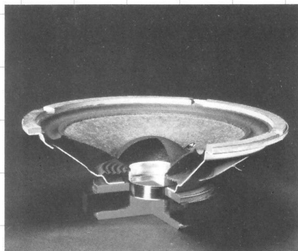
Schnittmodell des Tieftöners HD 306
