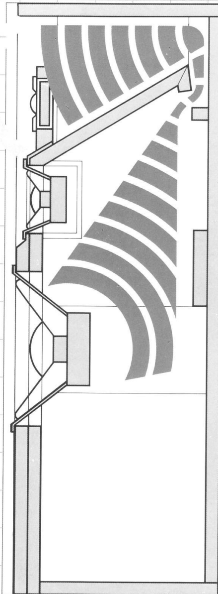
Hornresonatorprinzip Pat. Nr. P.2801227.3
