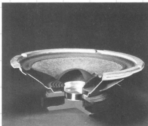
Schnittmodell des Tieftöners HD 306
