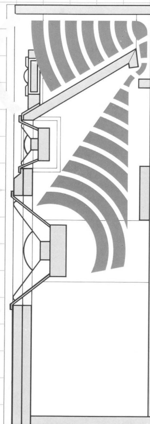
Hornresonatorprinzip Pat. Nr. P.280.1227.3
