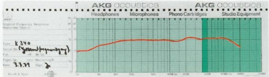
Frequenzkurve gesamt
