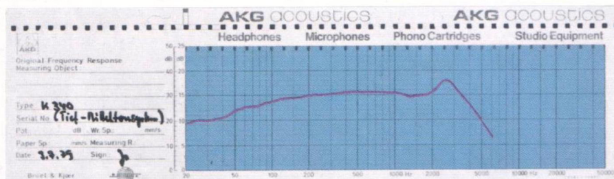
Frequenzkurve Tieftonsystem (dynamisch)
