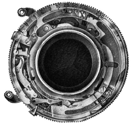
Compur-Verschuß geöffnet s. auch Abb. S. 4
