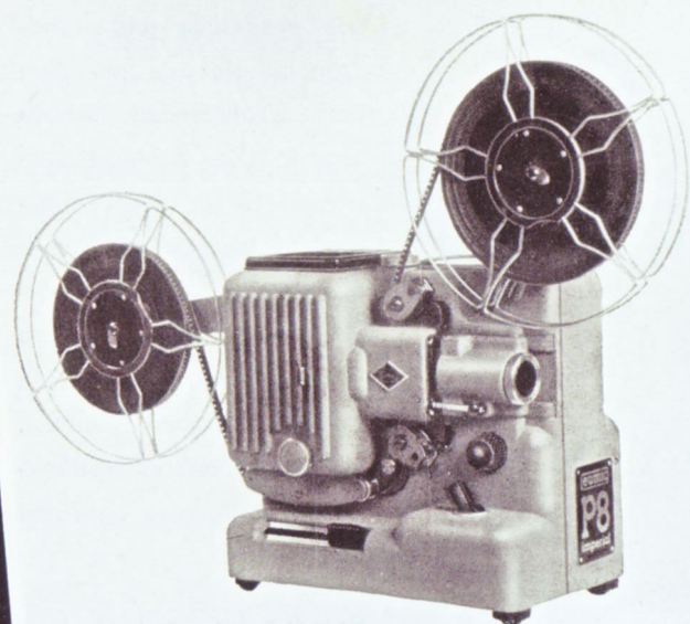
P 8 - Standard m. Lampe 100 W
