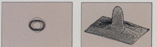
Meßcharakteristik Spotmessung
