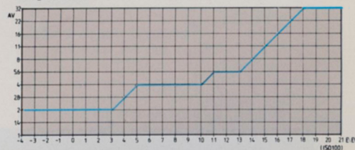
Programmkarakteristik bei Blitz-Meßwertspeicherung
