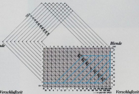
Charakteristik der Vario-Programmautomatik (mit FD 1:1,4/50 mm)
