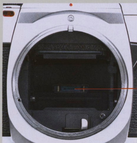
Hilfsspiegel
