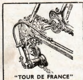
"SIMPLEX" TOUR DE FRANCE DERAILLEUR GEARS
