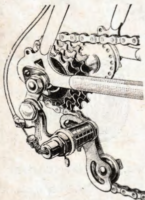
BENELUX DERAILLEUR GEARS
